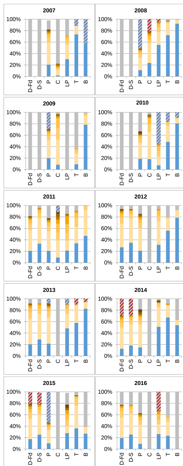
Figure 11 : Suivi de la concentration en matières en suspension en pourcentage de temps cumulé le long de l'estuaire, pour chaque année (réalisation : GIP Loire Estuaire - source des données : GIP Loire Estuaire)
