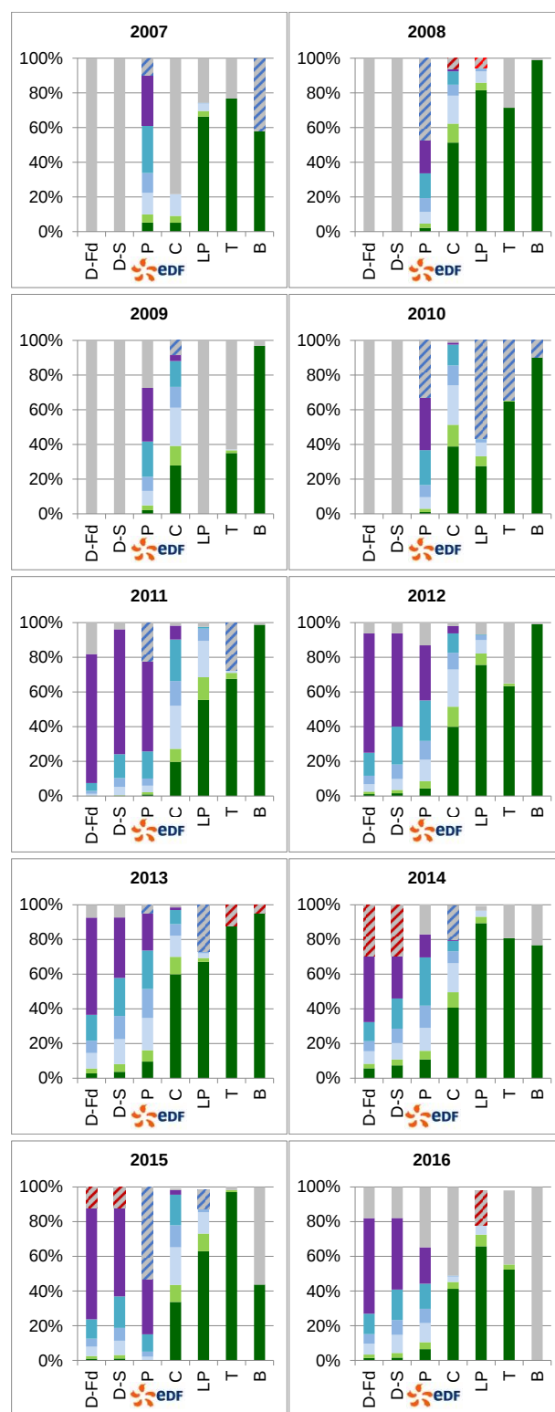
Figure 15 : Suivi de la salinité en pourcentage de temps cumulé le long de l'estuaire, pour chaque année (réalisation : GIP Loire Estuaire - sources des données : GIP Loire Estuaire, EDF)
