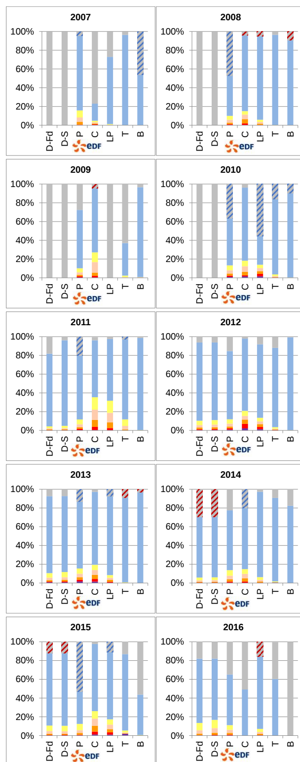
Figure 18 : Suivi de l'oxygène dissous en pourcentage de temps cumulé le long de l'estuaire, pour chaque année (réalisation : GIP Loire Estuaire - sources des données : GIP Loire Estuaire, EDF)
