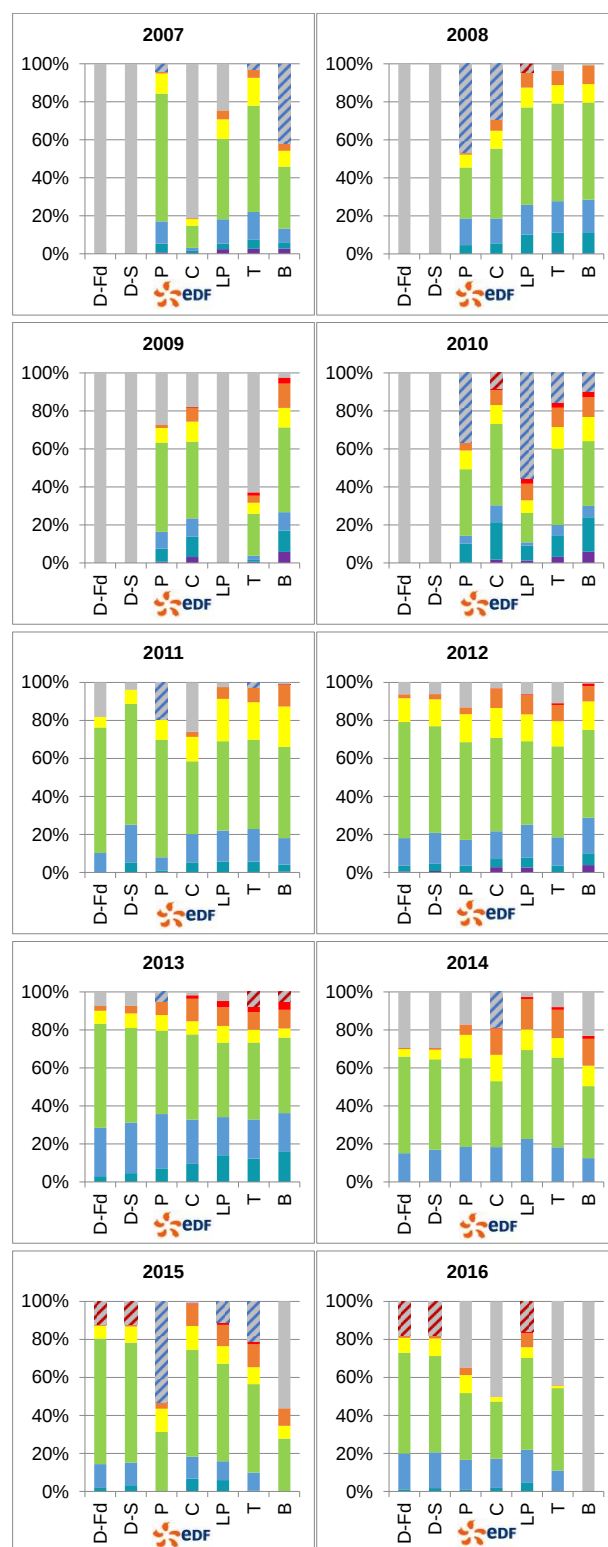
Figure 8 : Suivi de la température en pourcentage de temps cumulé le long de l'estuaire de la Loire, pour chaque année (réalisation : GIP Loire Estuaire - sources des données : GIP Loire Estuaire, EDF)
