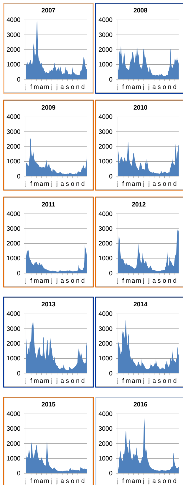
Figure 4 : Hydrogrammes 2007-2016 établis à partir des débits moyens journaliers en m 3 /s, à Montjean-sur-Loire (station située en secteur non soumis à la marée, à près de 112 kilomètres de l'embouchure) - Le contour coloré de chaque cadre se réfère à la figure 3 - (réalisation : GIP Loire Estuaire - source des données : DREAL Pays de la Loire)
