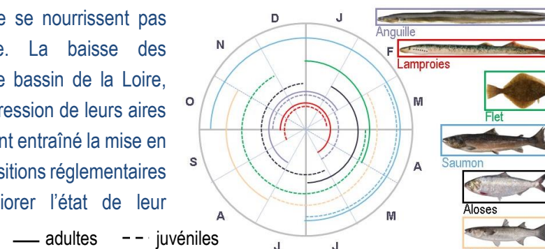
Figure 8 : périodes de passage des poissons migrateurs dans l'estuaire
