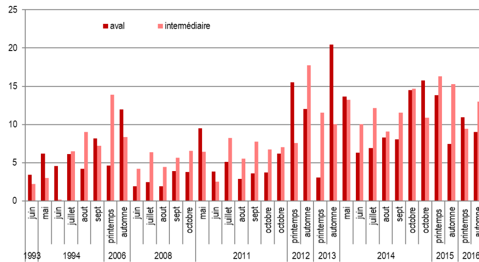
Figure 25 : biomasses par inventaire et par secteur entre mai et octobre depuis 1993
