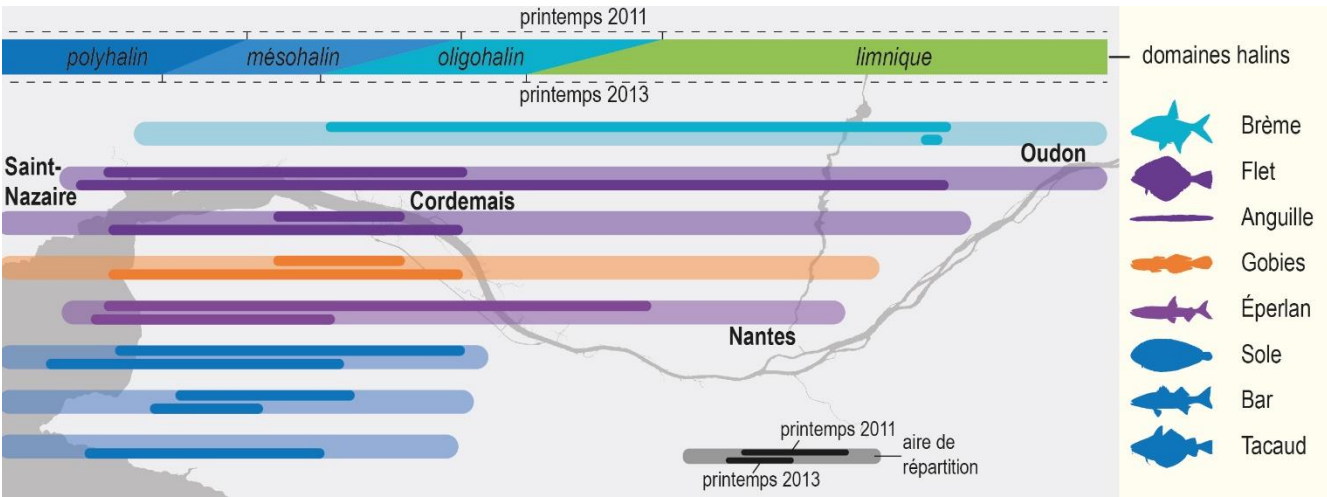
Figure 13 : aire de répartition maximale des espèces les plus fréquentes lors des inventaires des printemps 2011 (149 m³/s) et 2013 (1511 m³/s) avec les domaines halins correspondants
