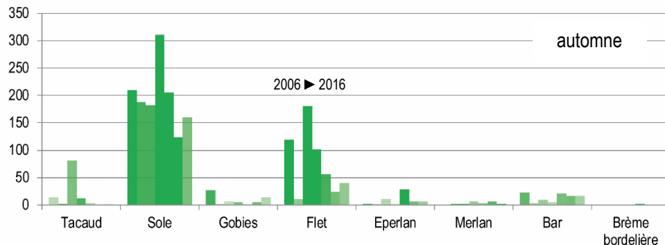
Figure 19 : densités des espèces principales (>20 ind/ha au moins une fois) dans les inventaires DCE (plus la fréquence est élevée, plus la couleur est foncée) - Source des données : AELB
