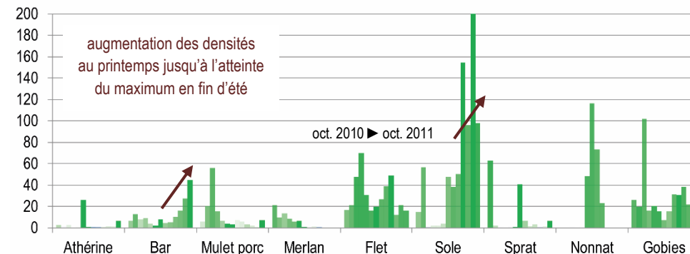
Figure 20 : densités des espèces principales (>20 ind/ha au moins une fois) dans l'inventaire d'octobre 2010 à octobre 2011 (plus la fréquence est élevée, plus la couleur est foncée) - Source des données : GPMNSN
