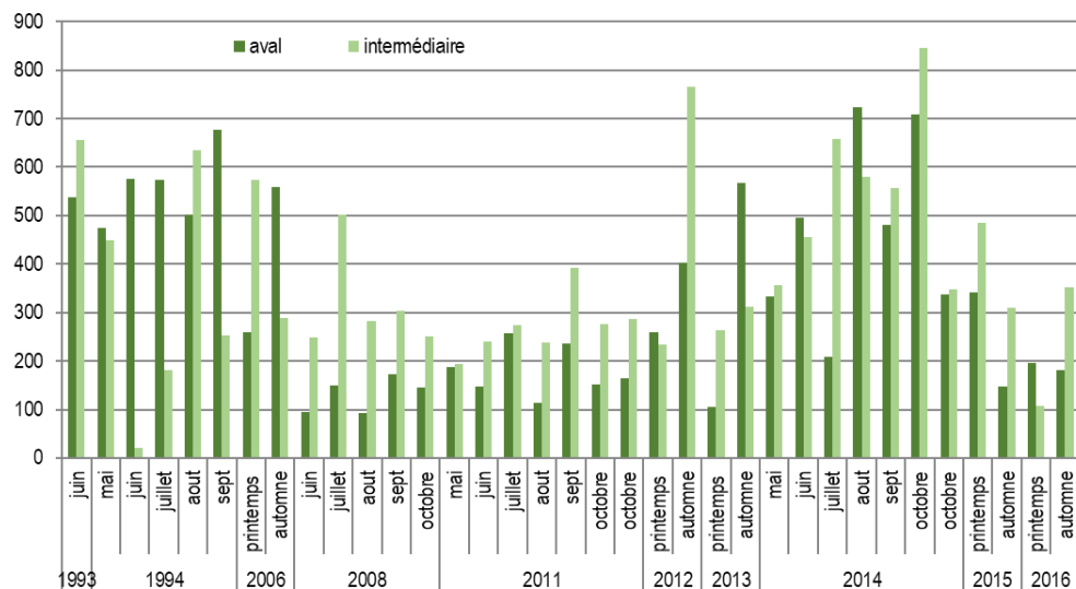
Figure 24 : densités par inventaire et par secteur entre mai et octobre depuis 1993 -
