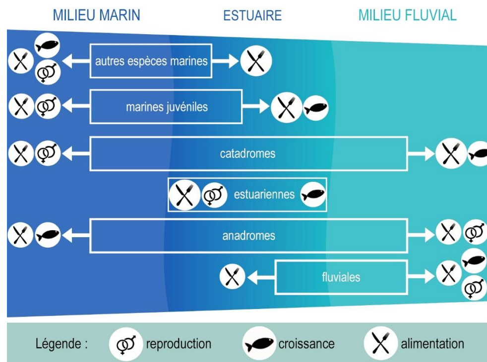
Figure 1 : représentation des 6 guildes écologiques présentes en estuaire
