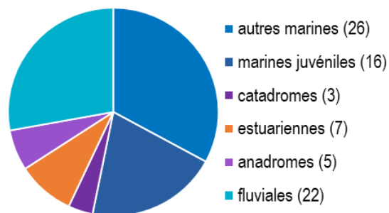
Figure 7 : répartition de la richesse spécifique par guildes - Sources des données : Université de Nantes, GPMNSN, GIP Loire Estuaire, Bio-Littoral, SMIDAP, AELB
