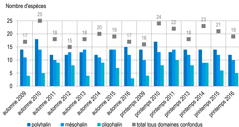
Figure 10 : richesses spécifiques par domaine halin et par inventaire - Source des données : AELB
