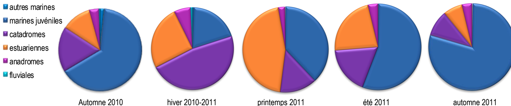
Figure 15 : abondances relatives (nombre d'individus/nombre total) par guildes écologiques sur une année, de 2010 à 2011 - Source des données : GPMNSN
