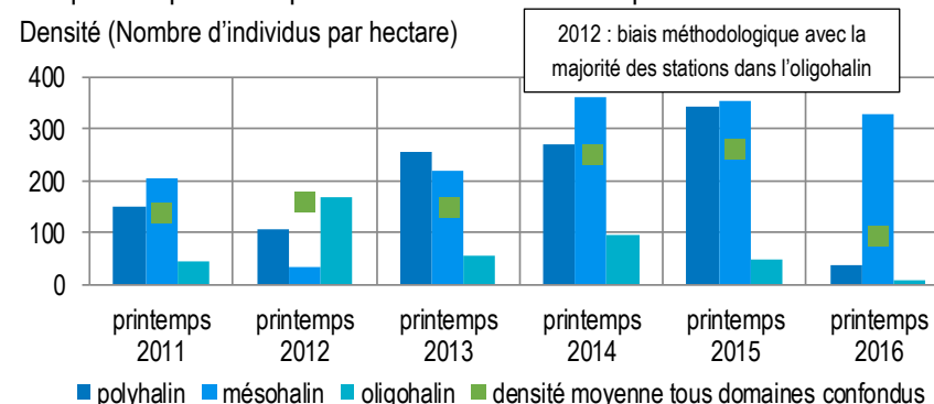
Figure 12 : densités moyennes et par domaine halin des inventaires DCE au printemps - Source des données : AELB
