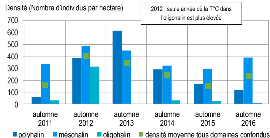
Figure 11 : densités moyennes et par domaine halin des inventaires DCE en automne - Source des données : AELB
