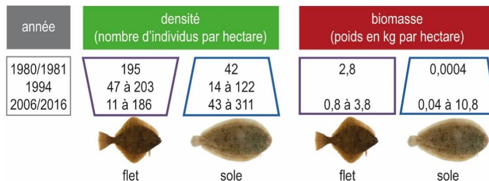
Figure 22 : densités et biomasses de flet et de sole entre 1980/1981 et 2006/2016
