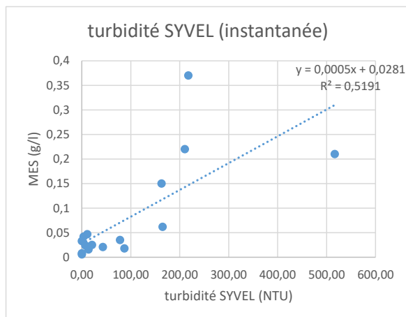
Figure 11 : Concentration en MES (g/l) en fonction de la turbidité instantanée (NTU) mesurée par la sonde SYVEL, sur la station de Bellevue
